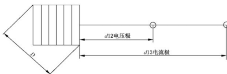
图 C.2 直线形布置
