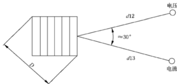
图 C.1 三角形布置
