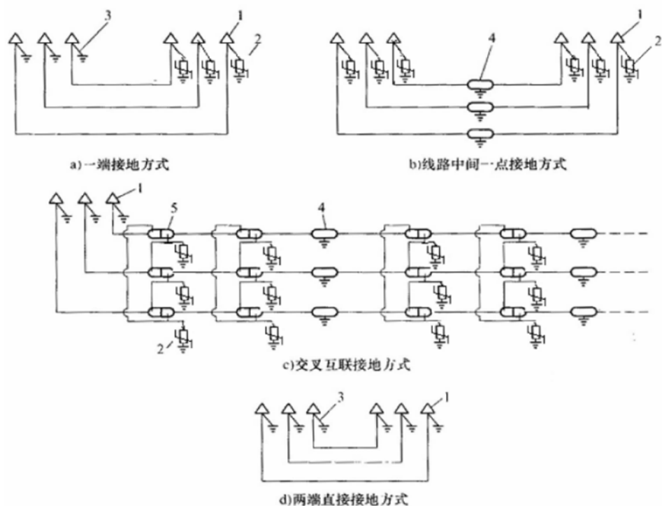
图 5.2.2 采用金属屏蔽层电压限制器时的接地方式
