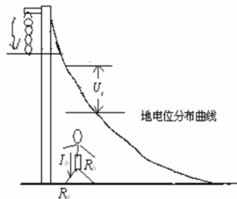
图7 人体遭受跨步电位差
