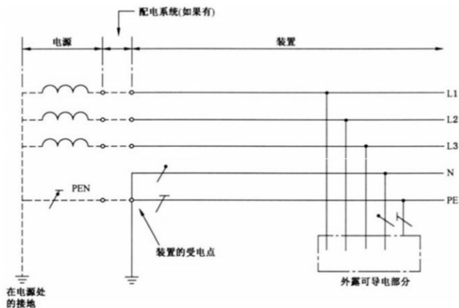
图 7.1.1-5 在装置的受电点将 PEN 分离成 PE 和 N 的 3 相 4 线制的 TN-C-S 系统
