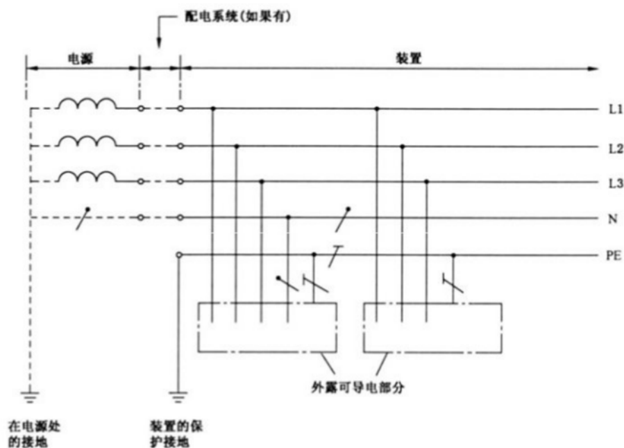
图 7.1.2-1 全部装置都采用分开的中性导体和保护导体的 TT 系统
