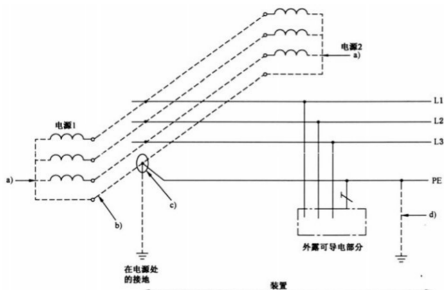
图 7.1.1-9 给 2 相或 3 相负荷供电的全系统内只有 PE 没有 N 的多电源 TN 系统
