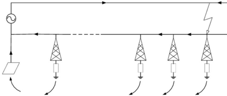
图 B.0.2-2 站外接地故障示意
