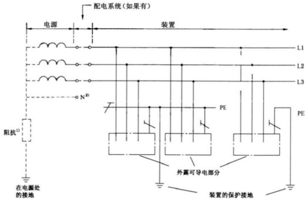
图 7.1.3-2 将外露可导电部分分组接地或独立接地的 IT 系统
