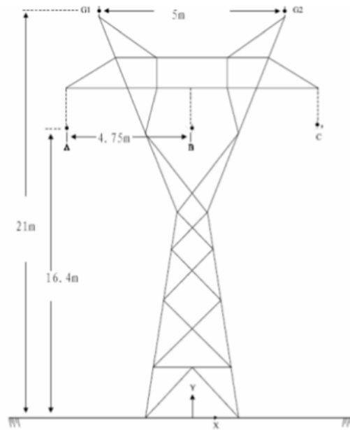
图 12 典型 110kV 型杆 SZ-16.4
