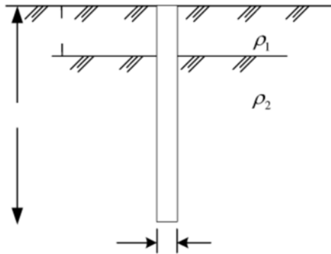
图 A.0.5-1 深埋接地体示意
