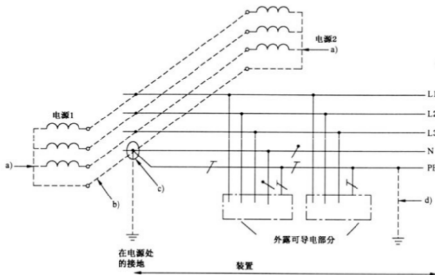
图 7.1.1-8 对用电设备采用单独的 PE 和 N 的多电源 TN-C-S 系统
