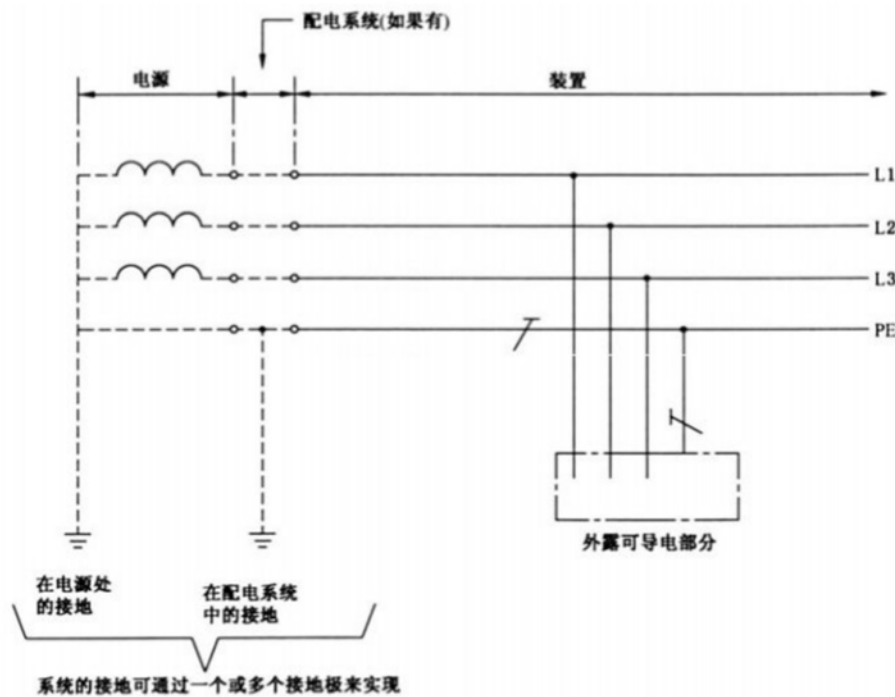
图 7.1.1-3 全系统采用接地的 PE 和未配出 N 的 TN-S 系统
