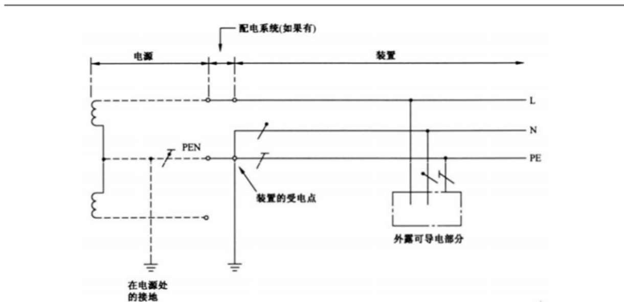
图 7.1.1-6 在装置的受电点将 PEN 分离成 PE 和 N 的单相 2 线制的 TN-C-S 系统
