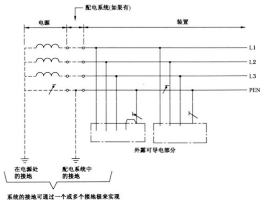
图 7.1.1-7 全系统采用将 N 的功能和 PE 的功能合并于一根导体的 TN-C 系统
