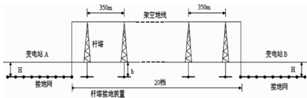
图 11 变电站 A 发生内部接地故障
