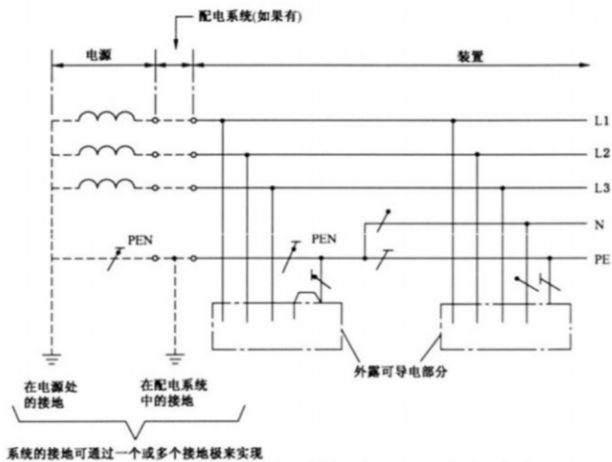
图 7.1.1-4 在装置非受电点的某处将 PEN 分离成 PE 和 N 的 3 相 4 线制的 TN-C-S 系统
