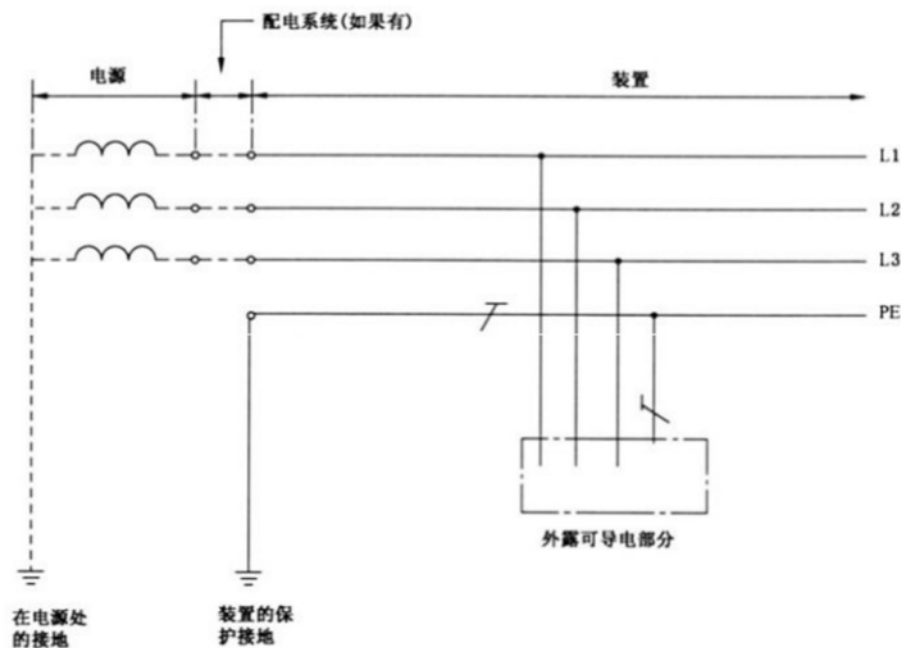
图 7.1.2-2 全部装置都具有接地的保护导体，但不配出中性导体的 TT 系统
