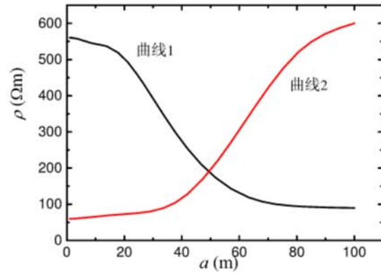
图2 双层土壤的典型视在电阻率曲线
