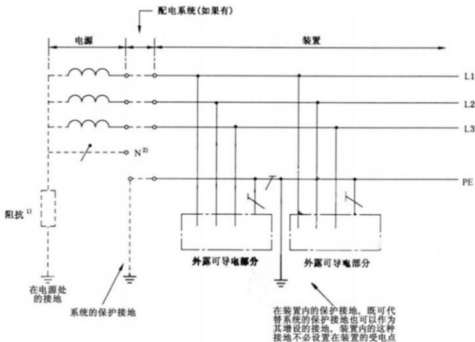
图 7.1.3-1 将所有的外露可导电部分采用 PE 相连后集中接地的 IT 系统
