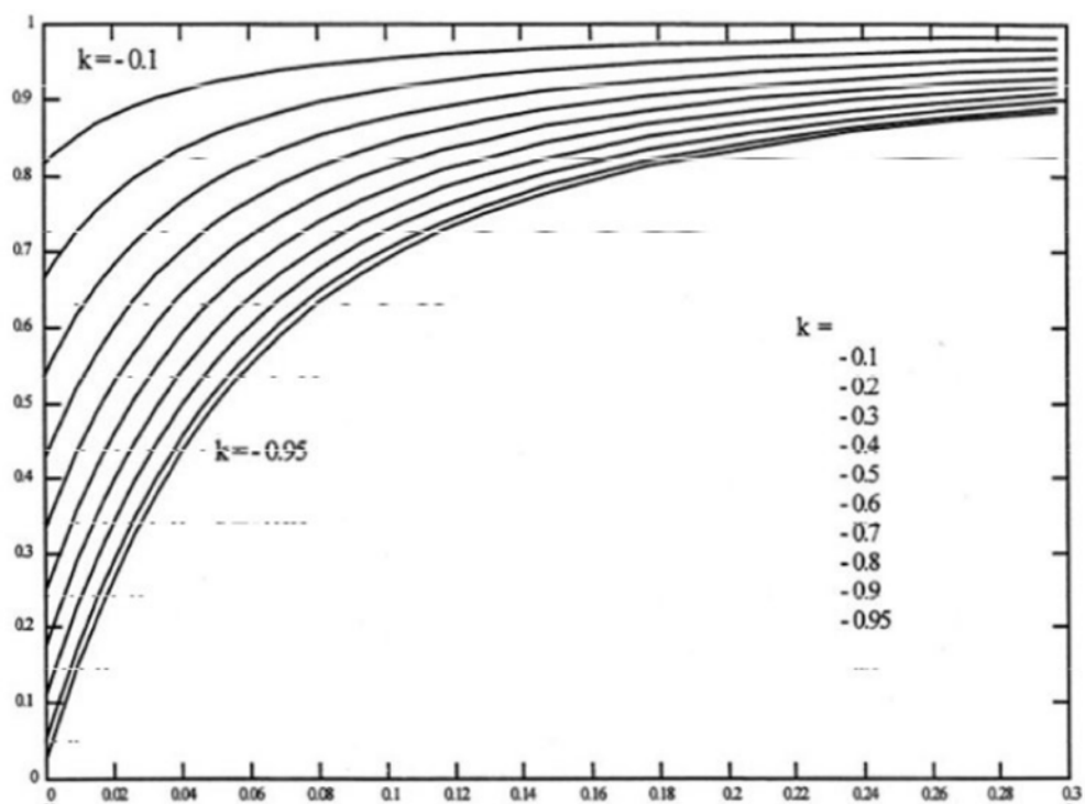
图 C.0.1 C_s 受 h 和 K 变化的曲线
