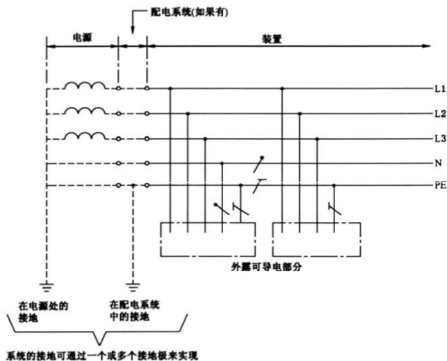
图 7.1.1-1 全系统将 N 与 PE 分开的 TN-S 系统
