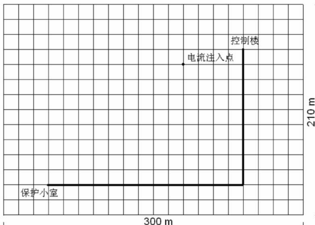
图 6 电缆和电流入地点的位置示意
