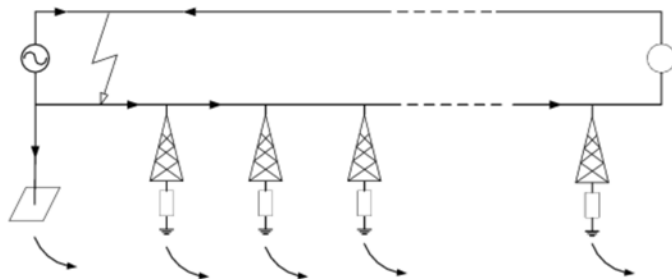
图 B.0.2-1 站内接地故障示意
