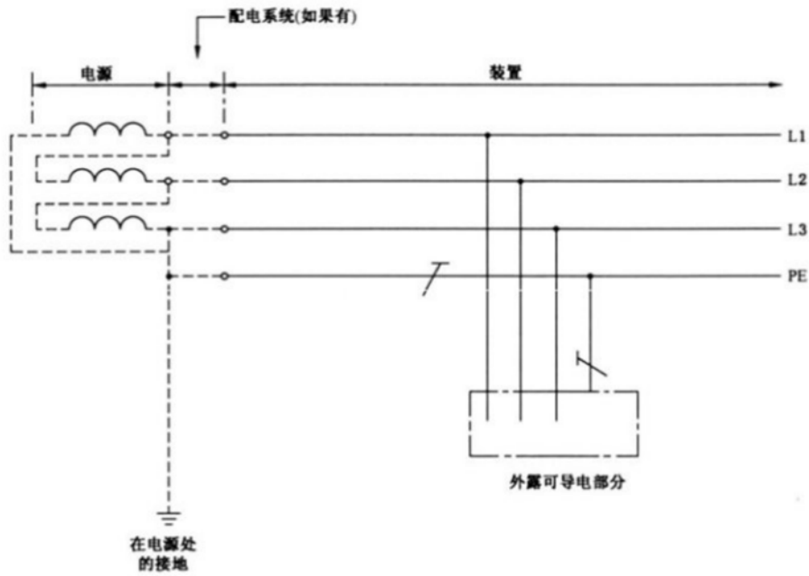
图 7.1.1-2 全系统将被接地的相导体与 PE 分开的 TN-S 系统
